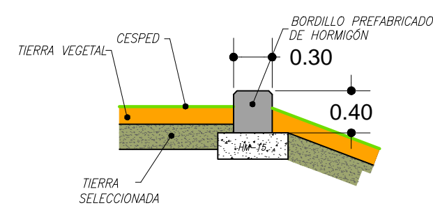
DETALLE 2
