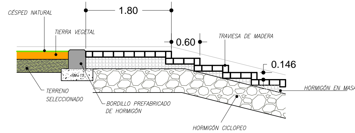
DETALLE 7
