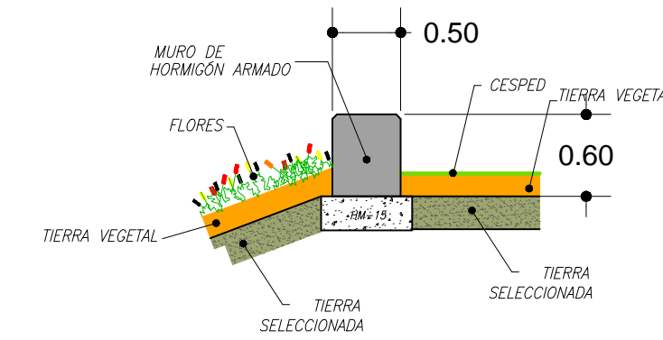
DETALLE 4
