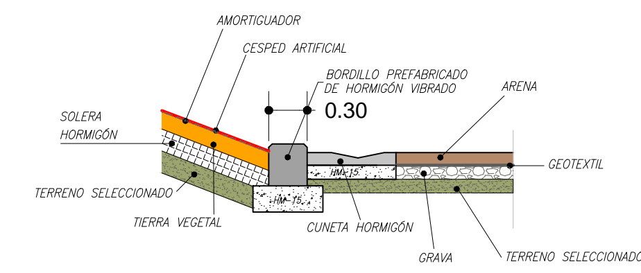
DETALLE 9
