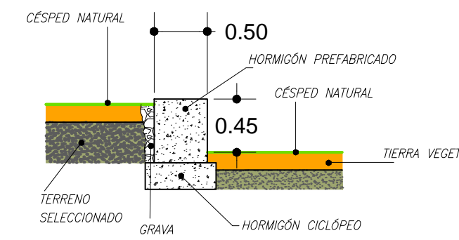
DETALLE 8
