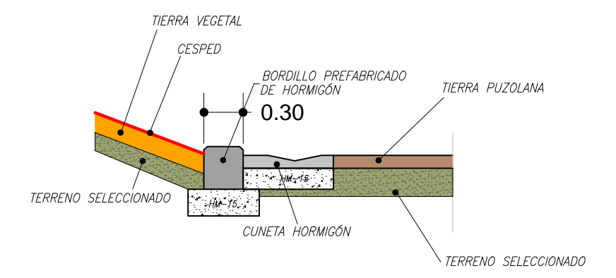
DETALLE 10
