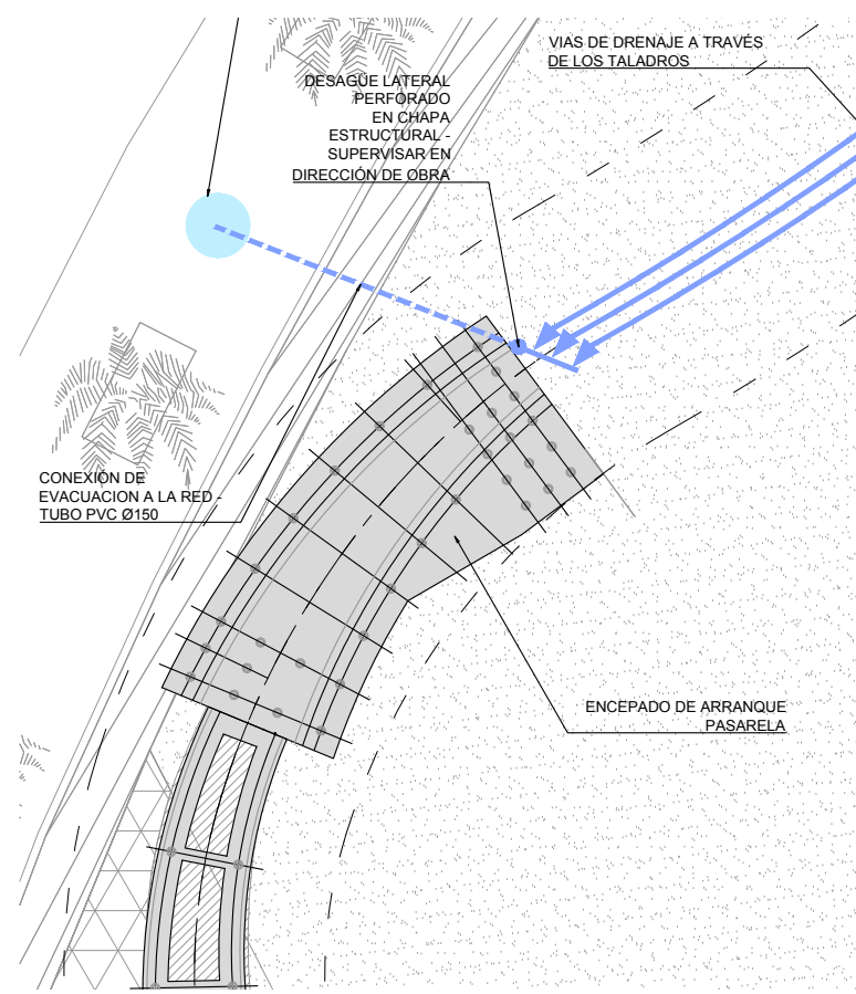
3 DETALLE RECOGIDA DEL DRENAJE EN MUELLE SANAPÚ I3.00 (A1) 1:100 / (A3) 1:200
