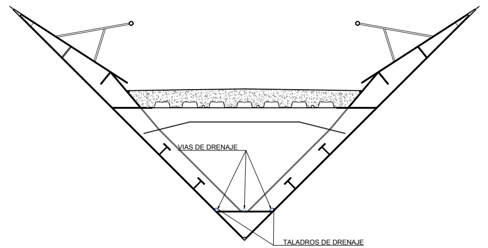
4 DETALLE SECCIÓN TRANSVERSAL I3.00 (A1) 1:25 / (A3) 1:50
