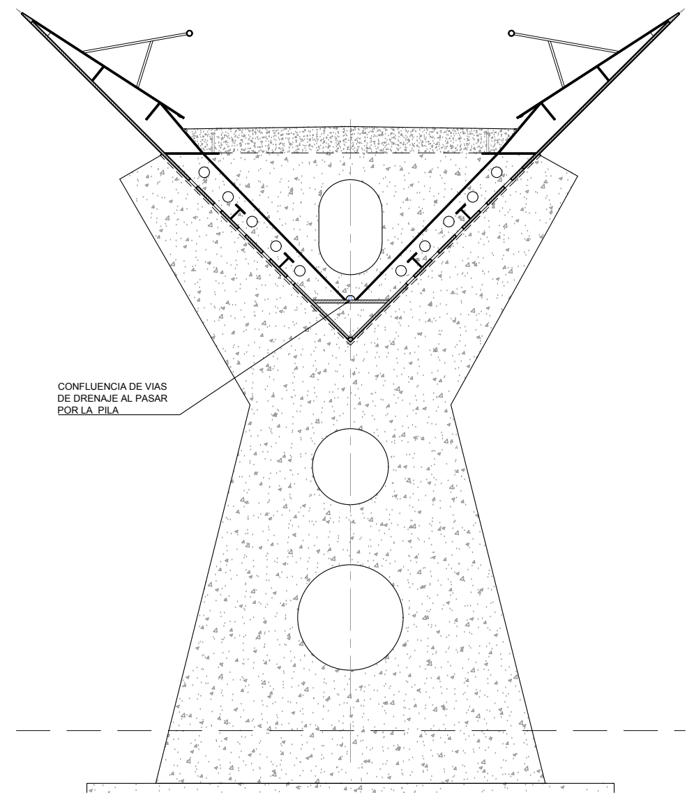
5 DETALLE SECCIÓN TRANSVERSAL EN PILA I3.00 (A1) 1:25 / (A3) 1:50
