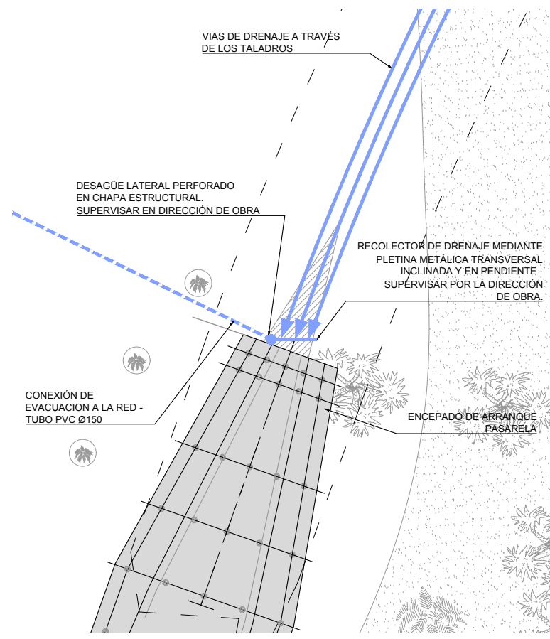
2 DETALLE RECOGIDA DEL DRENAJE EN MERCADO DEL PUERTO I3.00 (A1) 1:100 / (A3) 1:200
