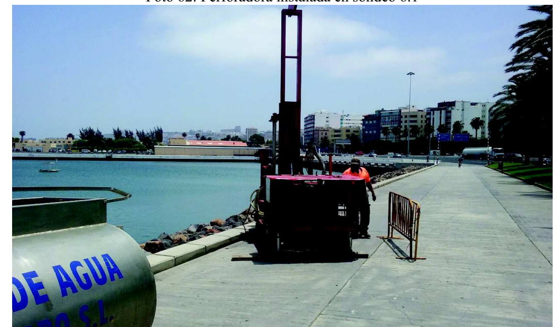
Foto 62: Perforadora instalada en sondeo 6.1
